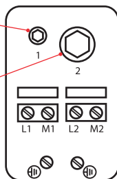
Электрическая схема
